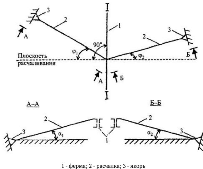
Рисунок К.2. Схема раскрепления ферм расчалками
