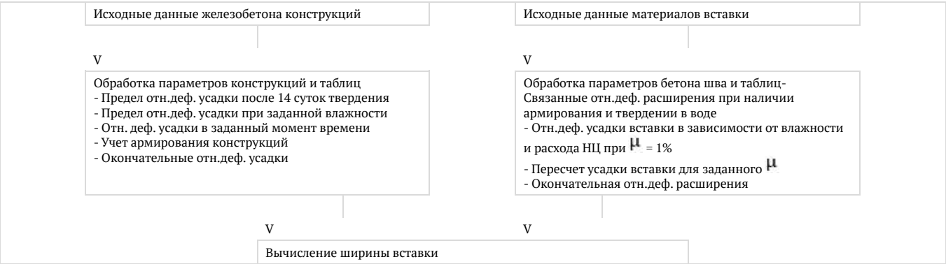
Схема вычислений ширины вставок
